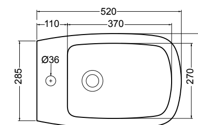
33020 bidet a terra_BTW bidet
