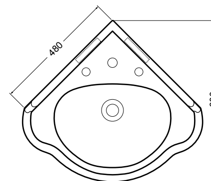
06035 lavabo angolo_corner basin
